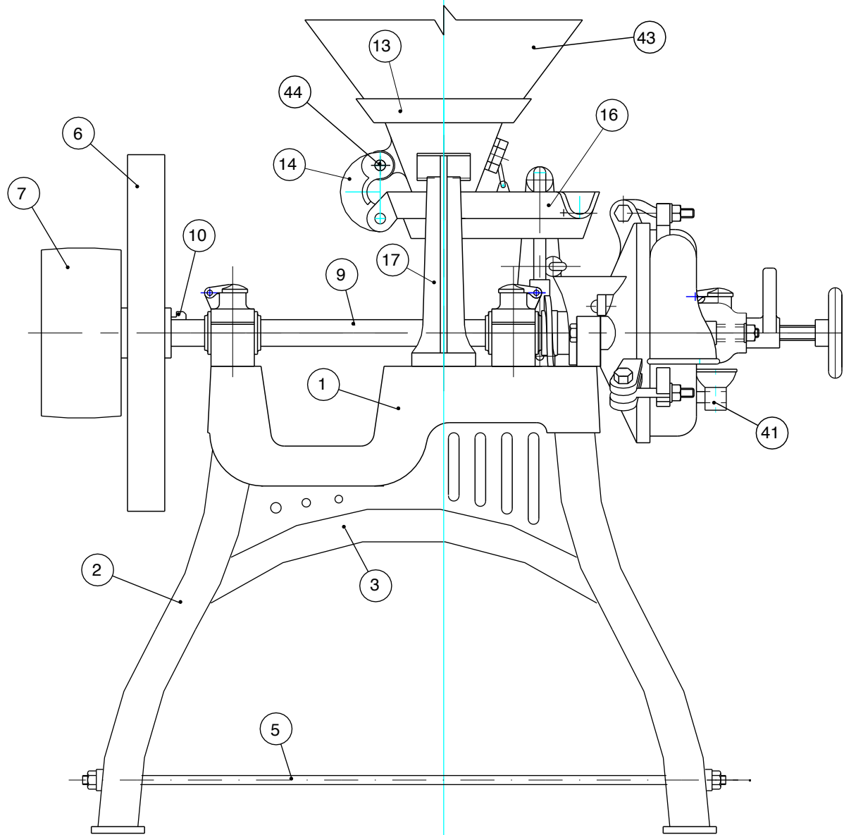
ELEVATION
