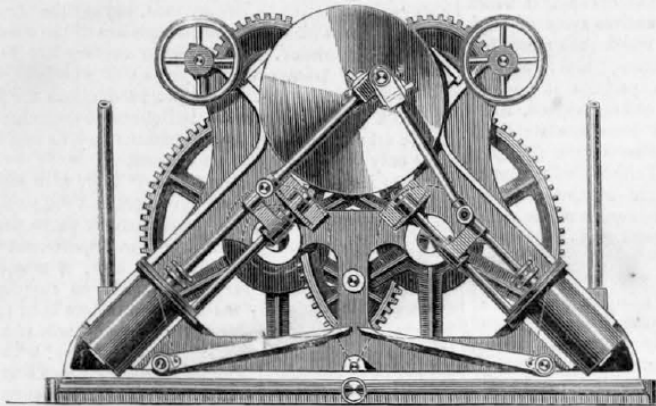
END ELEVATION
