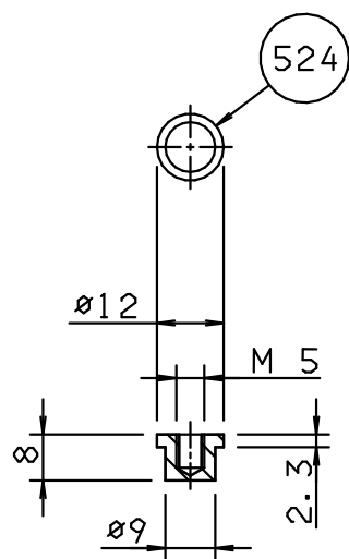
Blind Bush 1x
